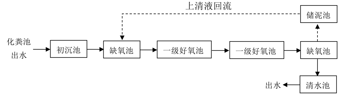
图 7.2-1 项目生活污水处理工艺流程示意图
