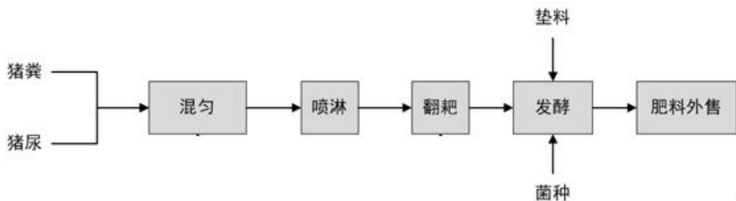
图 5-1 污水处理工艺图
