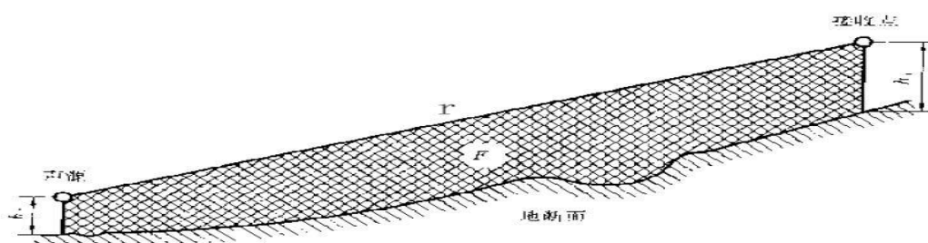
图4-7 估计平均高度 h_m 的方法
