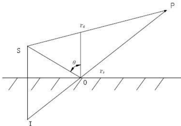
图 4-6 反射体的影响
