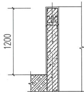
① 车道拦板详图1: 20
