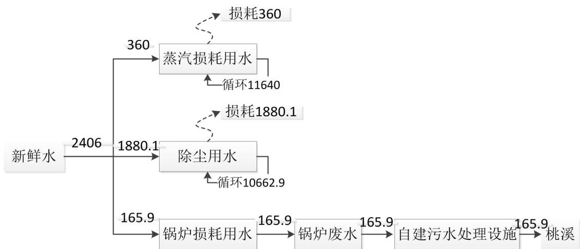
图 2.7-2 改建前项目水平衡图 单位 t/a
