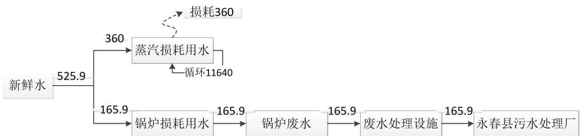
图 2.7-1 项目水平衡图 单位 t/a
