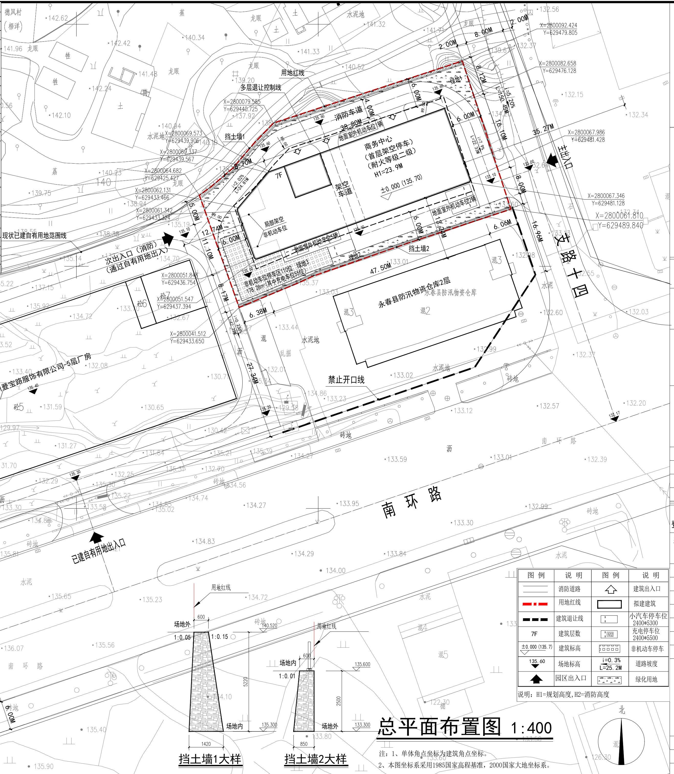
总平面布置图
