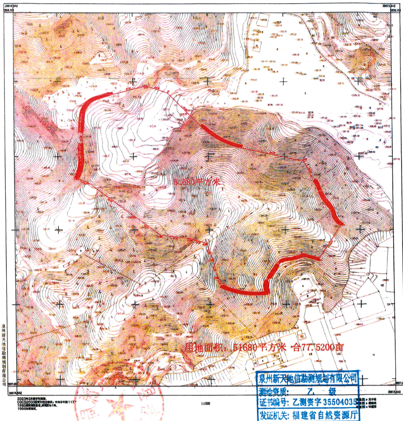
永春县2023-34号地块勘测定界图
